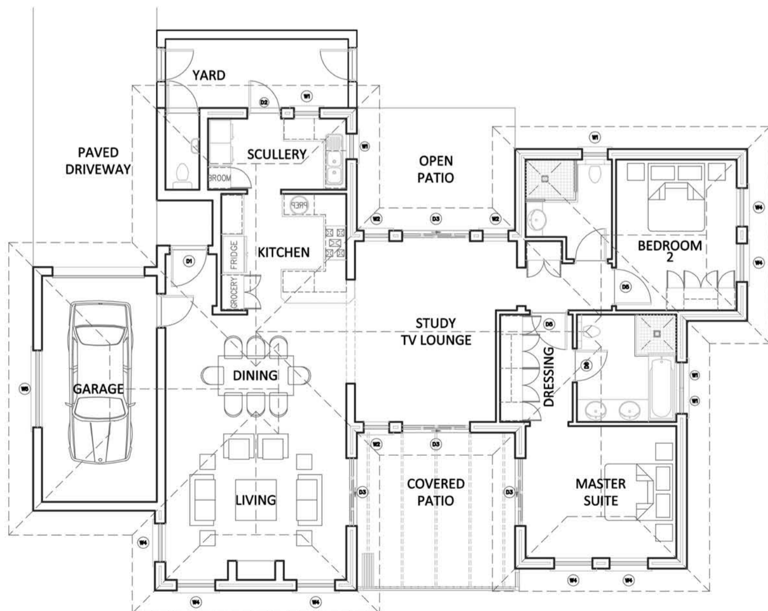
UNIT TYPE D1
